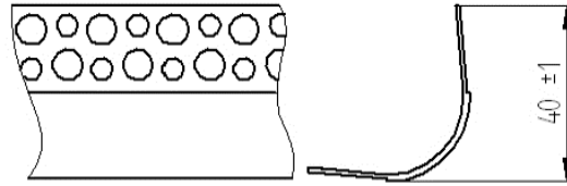
Fig. 20. Corner bead BP8
