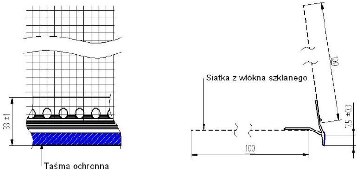
Fig. 3. Bead BP14 ECO PLUS
