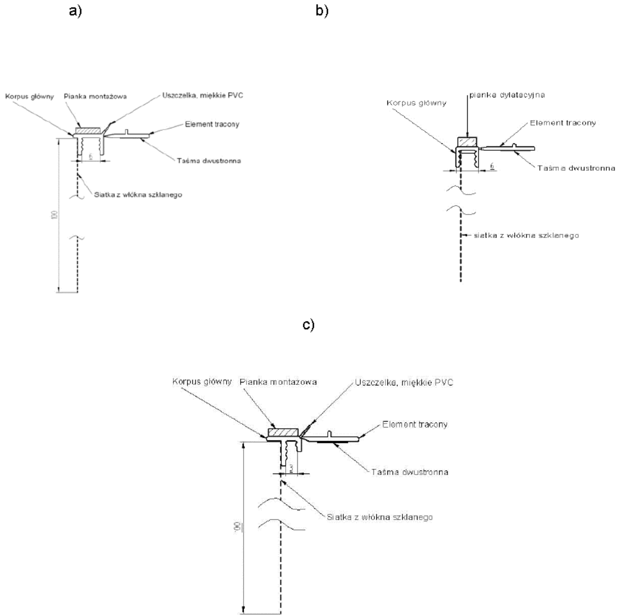
Fig. 1. Beads BP13 (a), BP13 MINI (b), BP13 MIDI (c)
