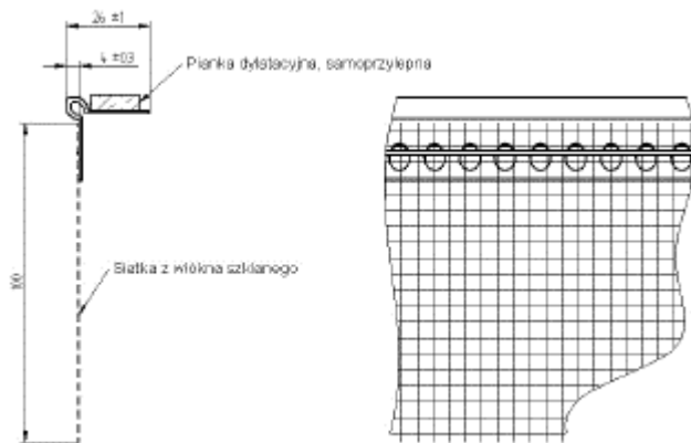
Fig. 9. Bead BP20
