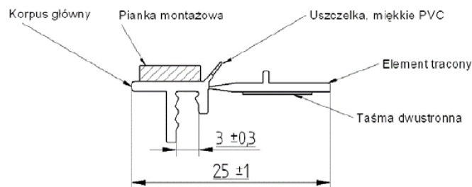
Fig. 22. Beads BP12 (a), BP12 MIDI (b), BP12 MINI (c)
