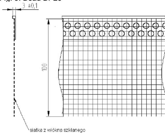
Fig. 10. Bead BP22
