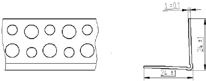
Fig. 16. Corner bead BP2
