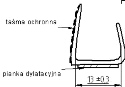
Fig. 19. Bead BP5
