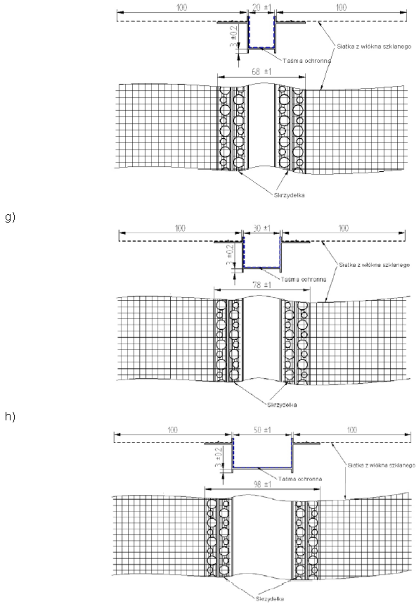
Fig. 6. Beads BP11 H1S (a), BP11 H2S (b), BP11 H3S (c), BP11 H3 NS (d), BP11 H5S (e), BP11 H2 RS (f), BP11 H3 RS (g), BP11 H5 RS (h)
