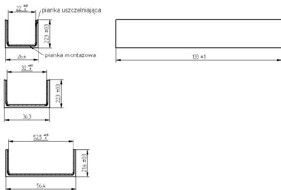
Fig. 12. Connectors BP11 Ł H1 (a) and BP11 Ł H2, BP11 Ł H3, BP11 Ł H5 (b)
