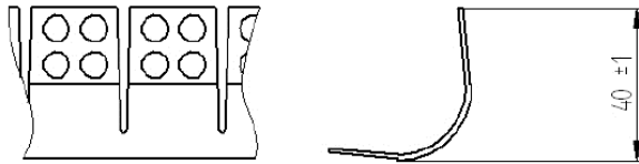
Fig. 21. Corner bead BP9
