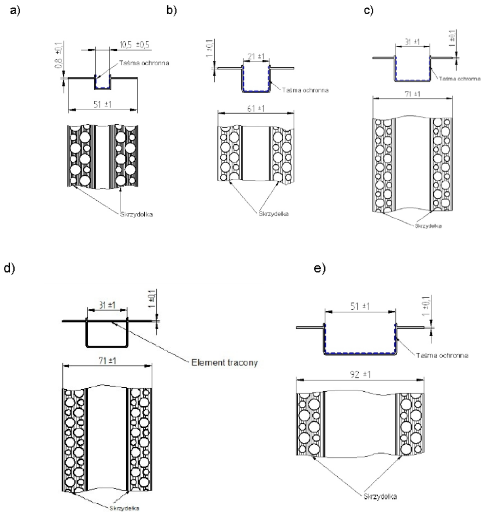
Fig. 4. Beads BP11 H1(a), BP11 H2 (b), BP11 H3 (c), BP11 H3N (d), BP11 H5 (e)
