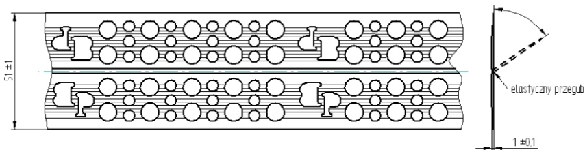
Fig. 18. Corner bead BP4
